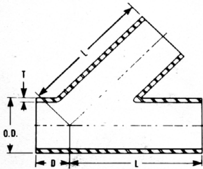
A28WA Lateral
