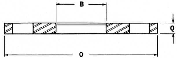
A38SL Flange
